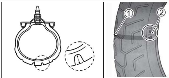
① 磨损指示标记 ② 磨损指示标记位置标识
